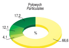
STRUKTURA ZANIECZYSZCZEŃ Z ZAKŁADÓW SZCZEGÓLNIIE UCIAŹLIWYCH W 2012 R. STRUCTURE OF POLLUTANTS FROM PLANTS ESPECIALLY NOXIOUS IN 2012
