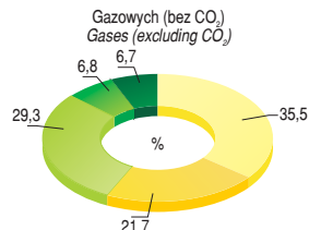
STRUKTURA ZANIECZYSZCZEŃ Z ZAKŁADÓW SZCZEGÓLNIIE UCIAŹLIWYCH W 2012 R. STRUCTURE OF POLLUTANTS FROM PLANTS ESPECIALLY NOXIOUS IN 2012
