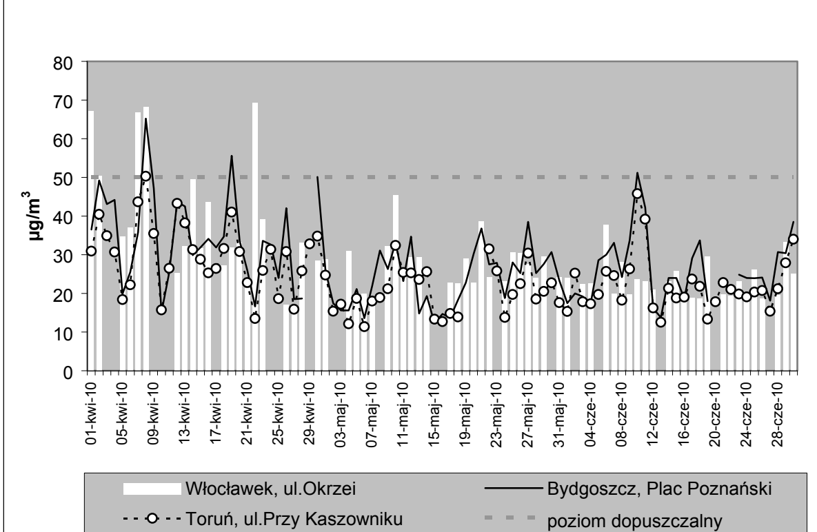
WYKRES 2 Stężenia 24-godzinne pyłu zawieszonego PM10 w II kwartale 2010 rok
