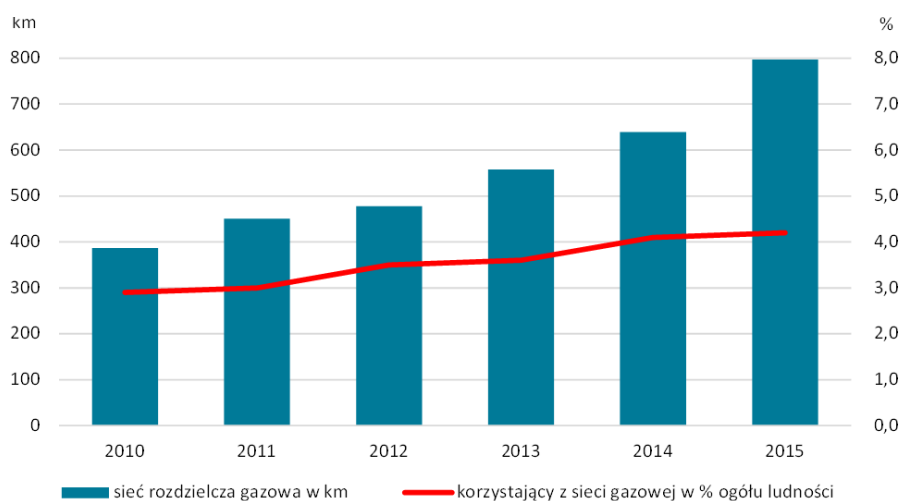
Wyk. 3. Sieć gazowa na obszarach wiejskich
